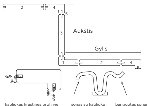
kabliukas kraštinės profilyje šonas su kabliuku banguotas šonas
